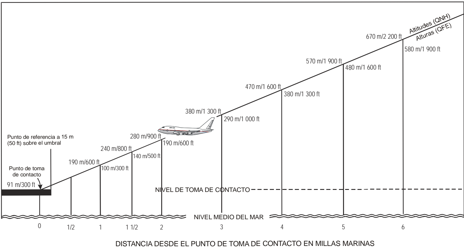
Figura 2. Aproximación con radar de vigilancia: Ejemplo de niveles para una trayectoria de plano de 3°, con punto de toma de contacto a una elevación de 300 ft AMSL
