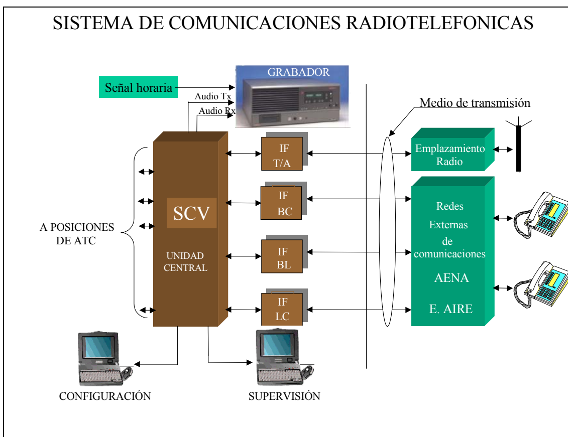
Figura 3.1.- Diagrama de bloques de un SCV
